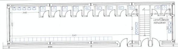
PLANTABAJA
