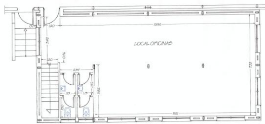
PLANTABAJA
