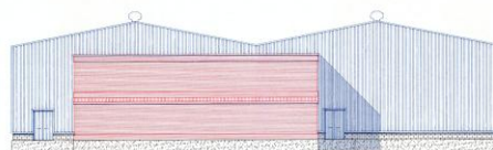
ALZADO POSTERIOR
